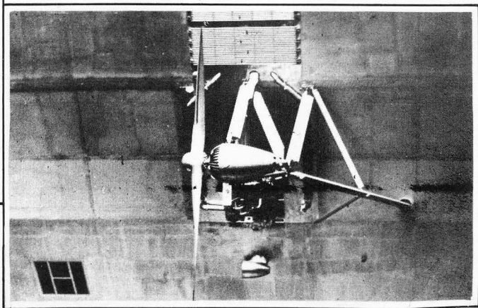
Detalle de una de las hélices reversibles del "Akron". Los motores están dentro del involucro. (Foto International).
