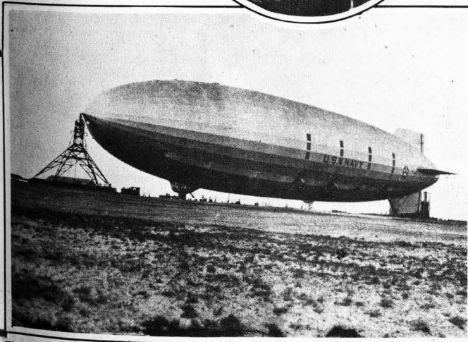
El "Akron" amarrado a su mástil en la base aérea de Lakehurst, antes de emprender su crucero por el Caribe. (Foto International).
