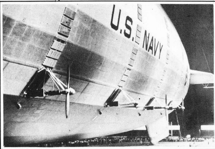
Cuatro de las ocho hélices propulsoras del "Akron". El gran dirigible pasó por La Habana moviéndose con dos máquinas de cada costado, a pequeña velocidad. (Foto International).
